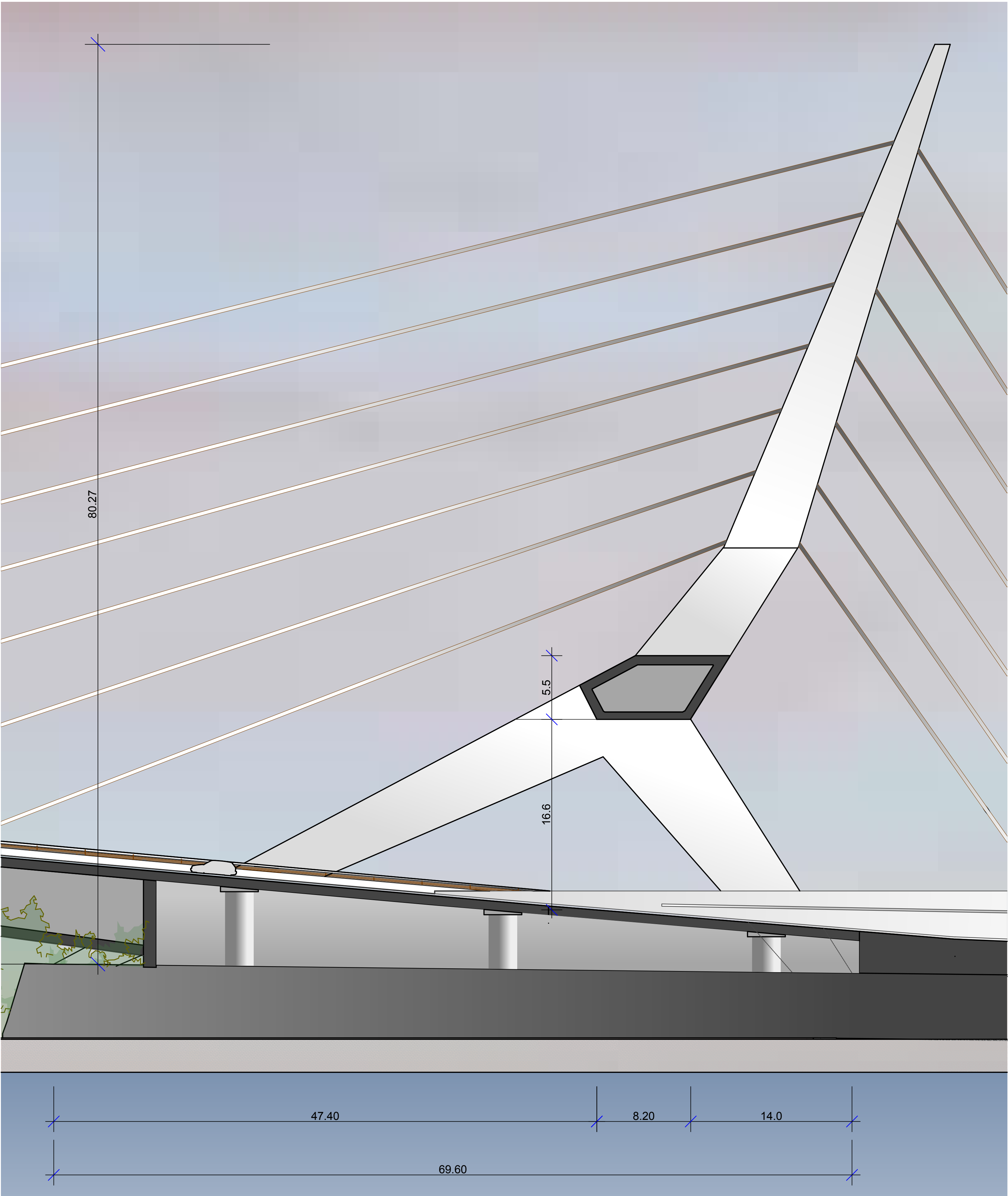
LONGITUDINAL SECTION
